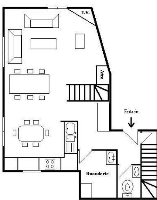
Niveau 1
